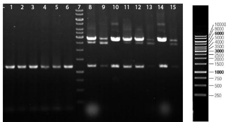
شکل ۲- الکتروفورز محصولات RT-PCR با استفاده از آغازگرهای ZYMV-8407-s و ZY3 (راهک‌های ۱ تا ۶) و پلاسمیدهای نو ترکیب حاوی ZYMV-CP ناحیه (راهک ۸ تا ۱۵) در ژل آگارز یک درصد. راهک ۷: مارکر GeneRuler 1 kb DNA Ladder.
