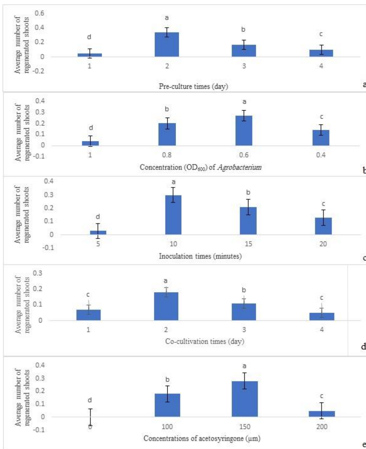
شکل ۳- (a) تاثیر زمان‌های مختلف پیش‌کشت (روز) بر میانگین تعداد شاخه‌های باززا شده در ریزنمونه‌های تراریخته، (b) تاثیر غلظت‌های مختلف OD_{600} آگروباکتریوم بر میانگین تعداد شاخه‌های باززا شده در ریزنمونه‌های تراریخته، (c) تاثیر زمان‌های مختلف تلقیح (دقیقه) بر میانگین تعداد شاخه‌های باززا شده در ریزنمونه‌های تراریخته، (d) تاثیر زمان‌های مختلف هم‌کشتی (روز) بر میانگین تعداد شاخه‌های باززا شده در ریزنمونه‌های تراریخته، (e) تاثیر غلظت‌های مختلف استوسیرینگون (میکرومولار) بر میانگین تعداد شاخه‌های باززا شده در ریزنمونه‌های تراریخته *حرف مشترک نشان دهنده عدم وجود اختلاف معنی‌دار در سطح احتمال ۵ درصد بر اساس آزمون دانکن می‌باشد
