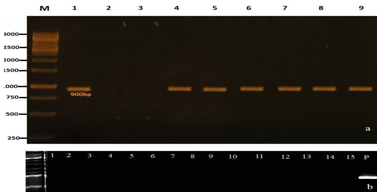
شکل ۵- a) الگوی الکتروفورزی محصولات PCR گیاهان تراریخت حاوی ژن کیتینازشیمیری با استفاده از آغازگرهای اختصاصی 35s و CHIT42R -M نشانگر وزن مولکولی (1 kb DNA ladder)، ۱- شاهد مثبت (قطعه تکثیر شده از پلاسمید حاوی ژن کیتیناز)، ۲- شاهد منفی (فاقد DNA)، ۳- شاهد منفی (محصول PCR از گیاه غیر تراریخت)، ۴ تا ۹- محصول PCR از گیاهان تراریخت. b) نتایج حاصل از واکنش زنجیره‌ای پلیمرز گیاهان تراریخته با استفاده از آغازگرهای اختصاصی ژن VirG -M نشانگر وزن مولکولی، ۱۰-۱۵ گیاهان تراریخت حاوی ژن کیتیناز، P: محصول PCR مربوط به آگروباکتریوم به عنوان شاهد مثبت
