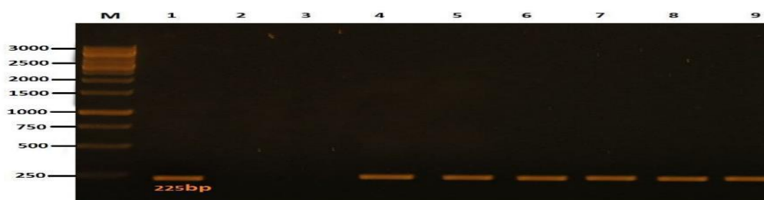
شکل ۶- a) الگوی الکتروفورزی محصولات PCR گیاهان تراریخت حاوی ژن کیتینازشیمیری با استفاده از آغازگرهای اختصاصی FchBD1 و RchBD -M نشانگر وزن مولکولی (1 kb DNA ladder)، ۱- شاهد مثبت (محصول PCR از سازه pBISM2)، ۲- شاهد منفی (فاقد DNA)، ۳- کنترل منفی (محصول PCR از گیاه غیر تراریخت)، ۴ تا ۹- محصول PCR از گیاهان تراریخت
