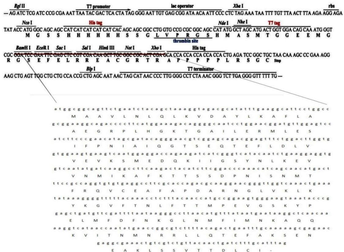
شکل ۴- محل‌های همساز سازی چندگانه مربوط به پلاسمید pET28a (+) در قسمت بالا و توالی نوکلئوتیدی به دست آمده از ژن پروتئین پوششی ویروس لکه برگ‌گی کروتیک سیب جدایه SSa در قسمت پایین، که توالی ژن با قسمت مشخص شده در MCS جایگزین گردید.
