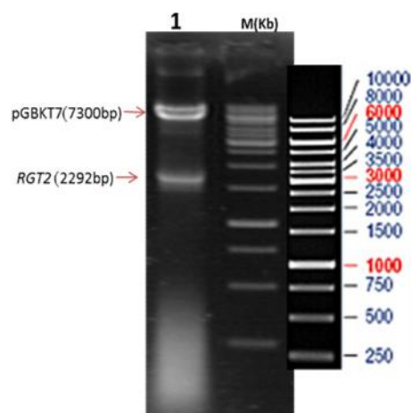
شکل ۷- تصویر الکتروفورز برش آنزیمی پلاسمید نو ترکیب (pGBKT7+RGT2) استخراج شده با آنزیم‌های PstI و NcoI . مشاهده‌ی باند ۲۲۹۲bp حضور فیزیکی قطعه همسانه‌سازی شده را تایید می‌کند. M(Kb) مارکر ۱kb.
