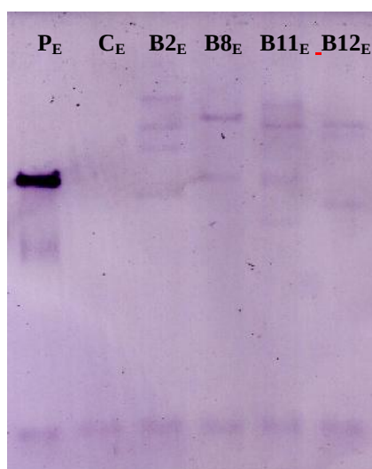
شکل ۳: تجزیه و تحلیل سادرن گیاهان تراریخته سیبزمینی حاوی ژن cry1Ab . PE، پلاسمید هضم شده با آنزیم EcoRI ، C_E گیاه غیرتراریخته هضم شده با آنزیم EcoRI ، B2_E ، B8_E ، B11_E ، B12_E به ترتیب گیاهان تراریخته لاین B2 ، B8 ، B11 و B12 هضم شده با آنزیم EcoRI .
