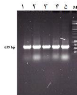
شکل ۲- تصویر الکتروفورز محصول واکنش زنجیره ای پلیمرز با آغازگرهای اختصاصی ژن merB روی دی ان ای استخراج شده از باکتری Serratia marcescens . باند ۶۳۹ جفت‌بازی با اندازه مورد انتظار برای ژن merB مطابقت داشت. ۱، ۲، ۳، ۴، ۵ تکرارهای مستقل هستند. (M: مارکر 1KB).
