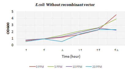
شکل ۱۰- تاثیر میزان متیل جیوه در محیط کشت روی رشد باکتری E.coli بدون وکتور نو ترکیب
