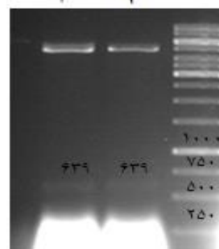
شکل ۵- تصویر الکتروفورز محصول هضم ژن merB با آنزیم‌های برشی NcoI و NdeI روی ژل آگارز. باند مربوط به ژن merB با اندازه ۶۳۹ جفت باز که با اندازه مورد انتظار برای ژن merB مطابقت داشت، از روی ژل جداسازی شد (M: مارکر 1KB).
