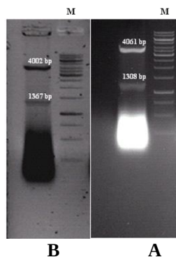
شکل ۳- تصویر الکتروفورز هضم وکتور PET-28a(+) با آنزیم‌های برشی روی ژل آگارز ۱٪: (الف) هضم وکتور با آنزیم‌های برشی SmaI و NdeI . (ب) هضم وکتور با آنزیم‌های برشی smaI و NcoI (M: مارکر 1KB).
