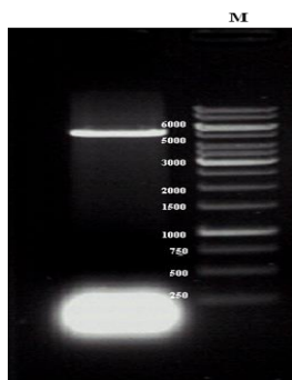
شکل ۴- تصویر الکتروفورز محصول برش آنزیمی وکتور pET-28a(+) توسط آنزیم‌های برشی NcoI و NdeI روی ژل آگارز ۱٪. جدا شدن وکتور خطی با اندازه حدود ۵۳۱۱ جفت باز با اندازه مورد انتظار برای وکتور pET-28a(+) مطابقت داشت (M: مارکر 1KB).
