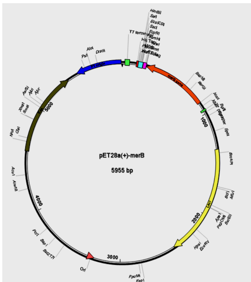
Figure 1- Constructed recombinant plasmid with merB gene. شکل ۱- شماتیک وکتور نو ترکیب ساخته شده حاوی ژن merB
