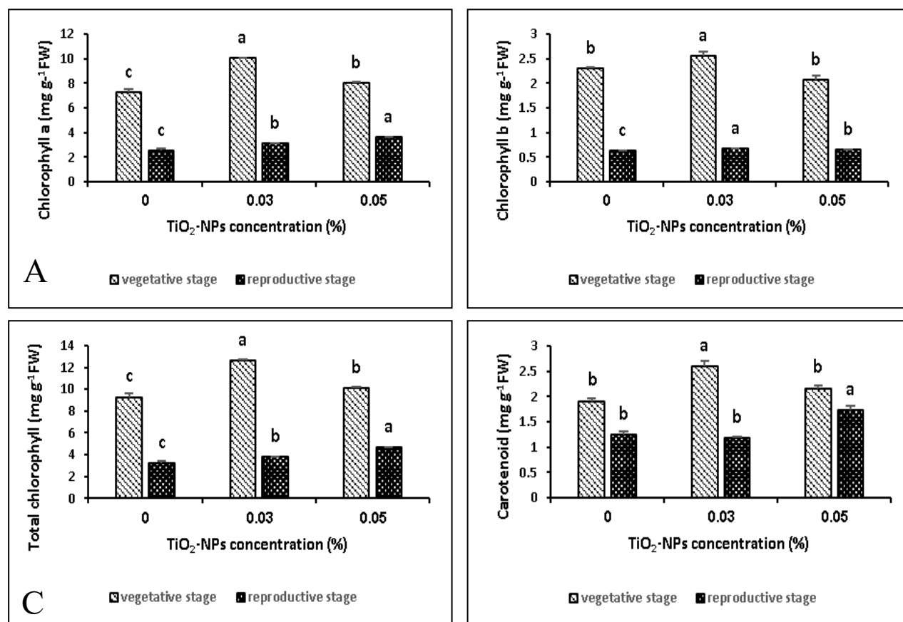
شکل ۴- اثر سطوح مختلف تیمار نانوذرات دی اکسید تیتانیوم بر رنگزه‌ها A: کلروفیل a، B: کلروفیل b، C: کلروفیل کل و D: کارتنوئید در مرحله رویشی و مرحله زایشی، در گیاه گل ناز یخی. حروف غیرمشابه بیانگر وجود اختلاف معنی‌دار در سطح احتمال ۰/۰۵ است.
