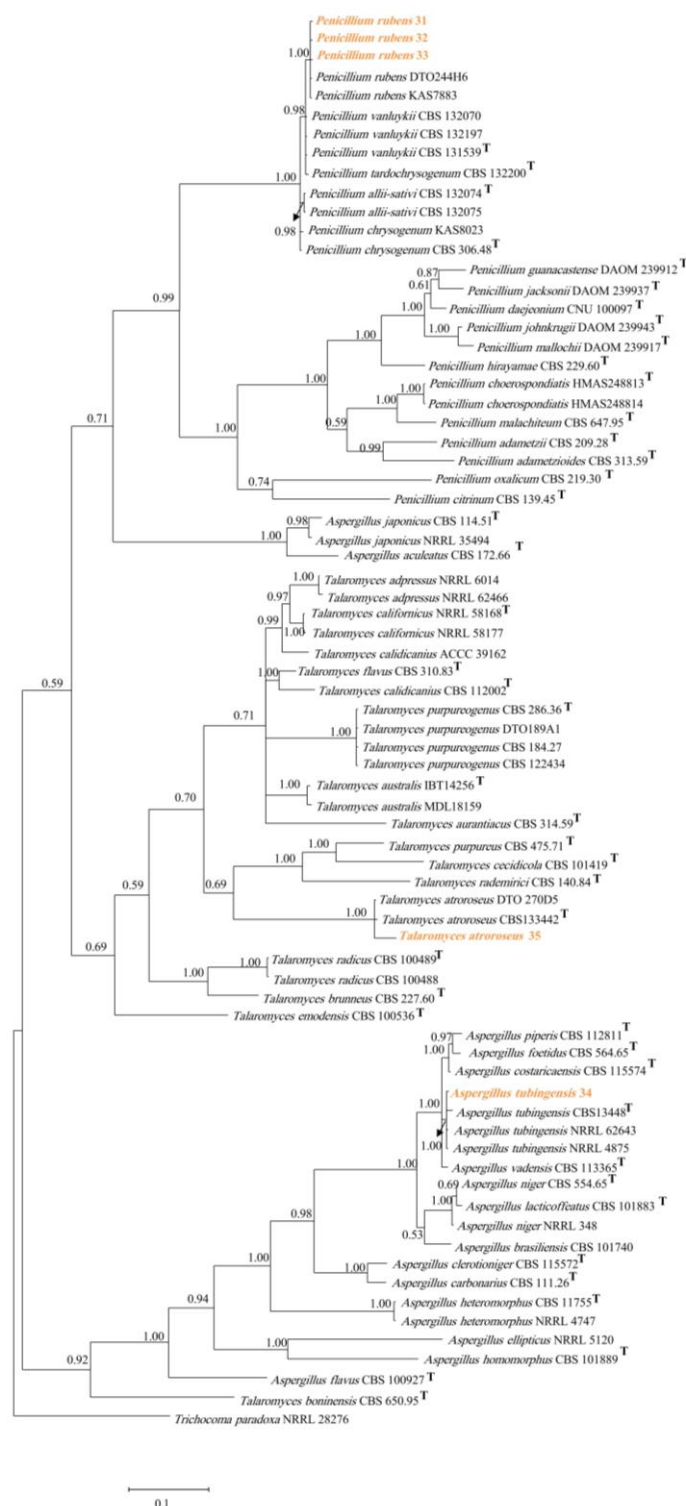
شکل ۲- استنتاج بیزی ناحیه \beta -tubulin برای جدایه‌های آسپرژیلوس و پنی‌سیلیوم با استفاده از نرم‌افزار MrBayes نسخه ۳.۱.۲.
