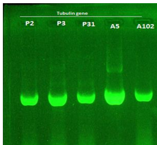
شکل ۱- الکتروفورز محصول PCR با آغازگرهای \beta -tubulin برای جدایه‌های آسپرژیلوس (A5) و پنی‌سیلیوم (P2, P3, P31, A102) در ژل آگاروز (۱٪).
