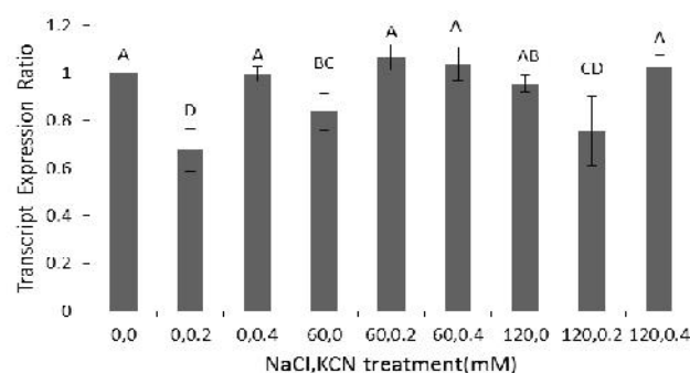
AdoMet S.
