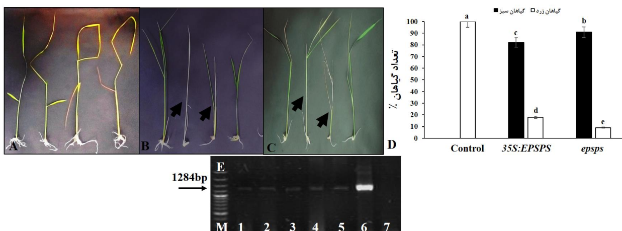
شکل ۴- بررسی گیاهان برنج تراریخته نسل دوم در محیط کشت انتخابی جامد حاوی جنتامایسین. (A) گیاهان شاهد، (B) گیاهان حاوی ژن 35S:EPSPS و (C) گیاهان حاوی ژن EPSPS . (D) درصد زنده‌مانی همان گیاهان در محیط کشت انتخابی حاوی جنتامایسین. گیاهان epsps تعداد گیاه سبزمان بیشتری در مقایسه با گیاهان 35S:EPSPS داشتند. (E) بررسی تعدادی از گیاهان تراریخته نسل دوم در واکنش PCR. (M) نشانگر، (۱ و ۲) گیاهان موتانت epsps ، (۳، ۴ و ۵) گیاه حامل ژن 35S:EPSPS (۶ کنترل مثبت و ۷ کنترل منفی).
