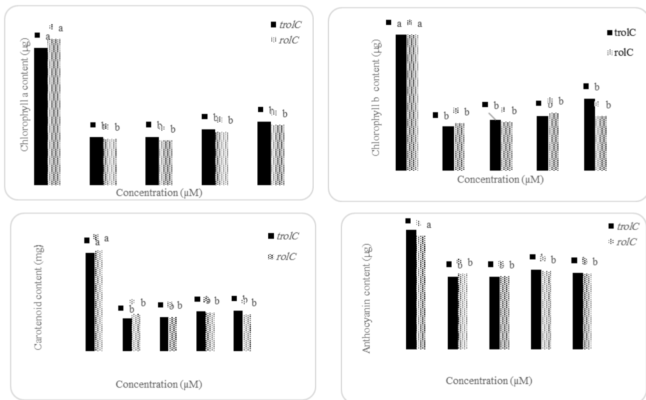
شکل ۲- محتوای رنگدانه‌های گیاهان تراژن rolC و trlC در تیمار با غلظت‌های فزاینده دگزامتازون (dex). دگزامتازون صفر \mu\text{M} شرایط شاهد را نشان می‌دهد.
