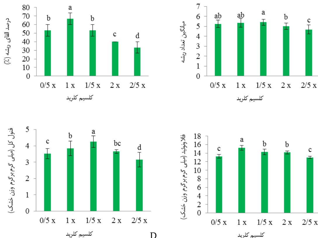
شکل ۴- تأثیر غلظت‌های مختلف کلسیم کلرید بر صفات ریشه‌های موین
