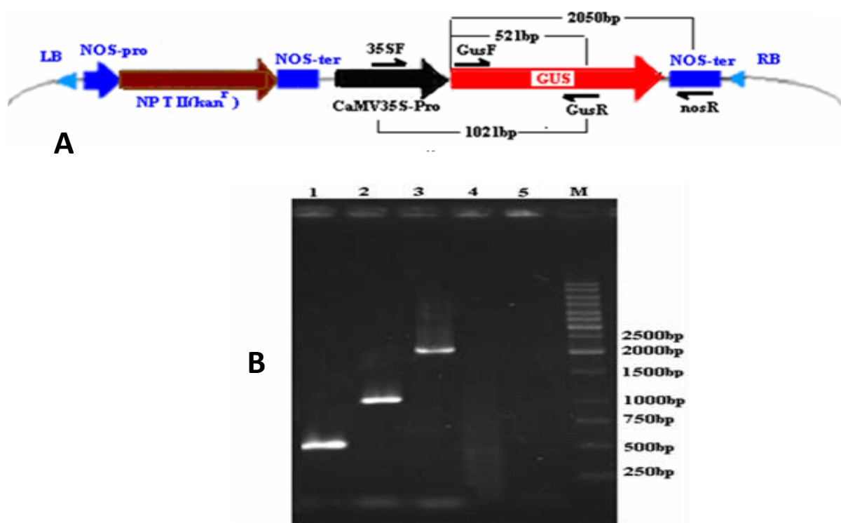
شکل ۲- A) شکل شماتیک پلاسمید pBI121^{GUS+} B) تأیید پلاسمید pBI121^{GUS+} توسط الگوی PCR در باکتری اگروباکتریوم (۱) محصول PCR با آغازگرهای (GusR/ GusF) (521bp)، (۲) محصول PCR با آغازگرهای (GusR /35sF) (1021 bp)، (۳) محصول PCR با آغازگرهای (nosR/GusF) (2050 bp)، (۴) محصول PCR با آغازگرهای (RbgnI/FbgnI) (0bp)، (۵) محصول PCR با آغازگرهای (RbgnI/35sF) (0bp)، (M) مارکر.
