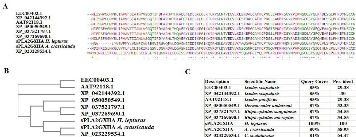
شکل ۴- توالی‌های پروتئینی ژن فسفولیپاز A2 ترشح شونده گروه XIIA مشتق شده از غده زهر عقرب H. lepturus همترازی توالی ۹ پروتئین sPLA2GXIIA مربوط به بندپایان مختلف (A)، درخت فیلوژنی (B) و مشخصات توالی‌های مربوط به آن‌ها (C) نشان داده شده است.
