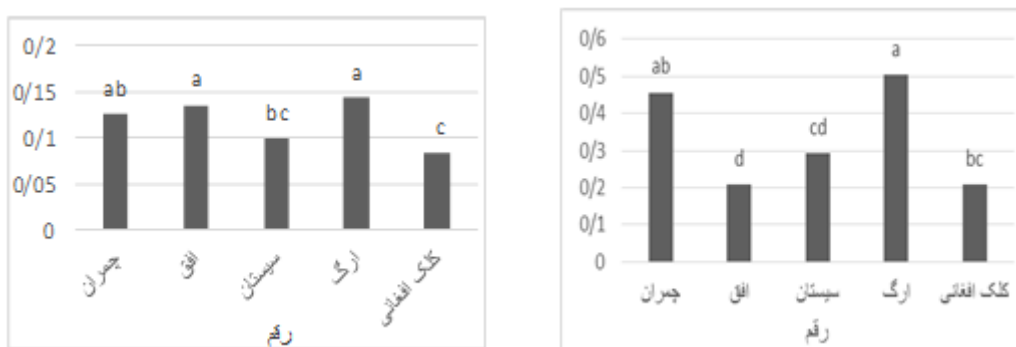
شکل ۱- میزان تغییرات فعالیت آنزیم کاتالاز (راست) و گایاکول پراکسیداز (چپ) در پنج رقم گندم نان تحت تنش خشکی.
