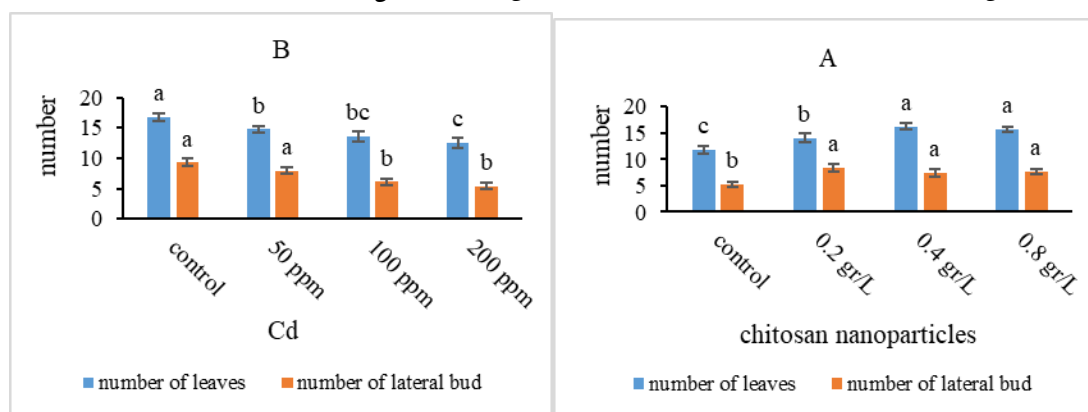
شکل ۳- مقایسه میانگین اثر ساده نانوذره کیتوزان (A) و اثر ساده کادمیوم (B) بر تعداد برگ و تعداد جوانه جانبی گیاه بادرنجبویه. حروف مشابه نشان‌دهنده عدم وجود اختلاف معنی‌دار می‌باشند.
